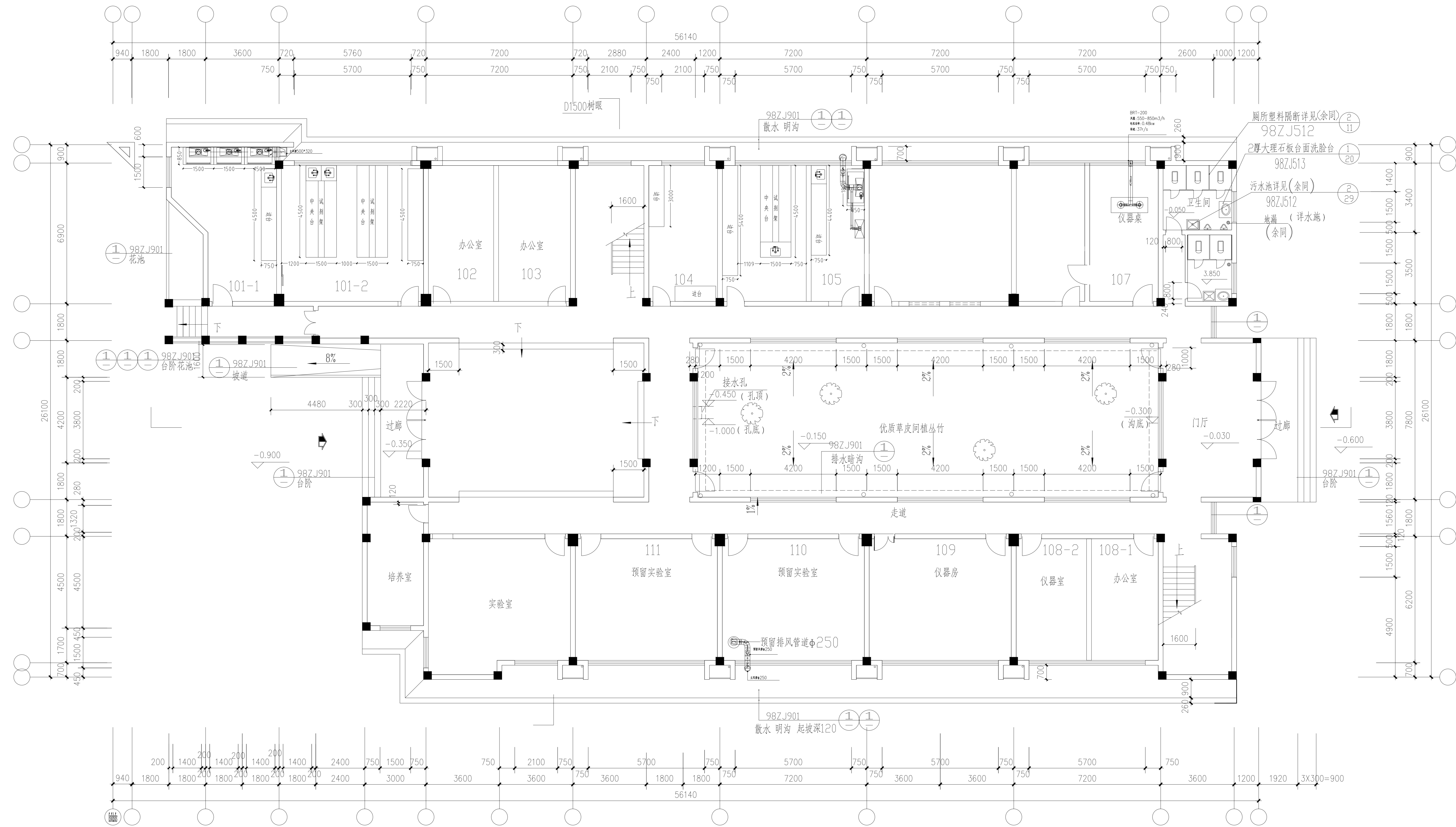
一层通风平面图1:100
