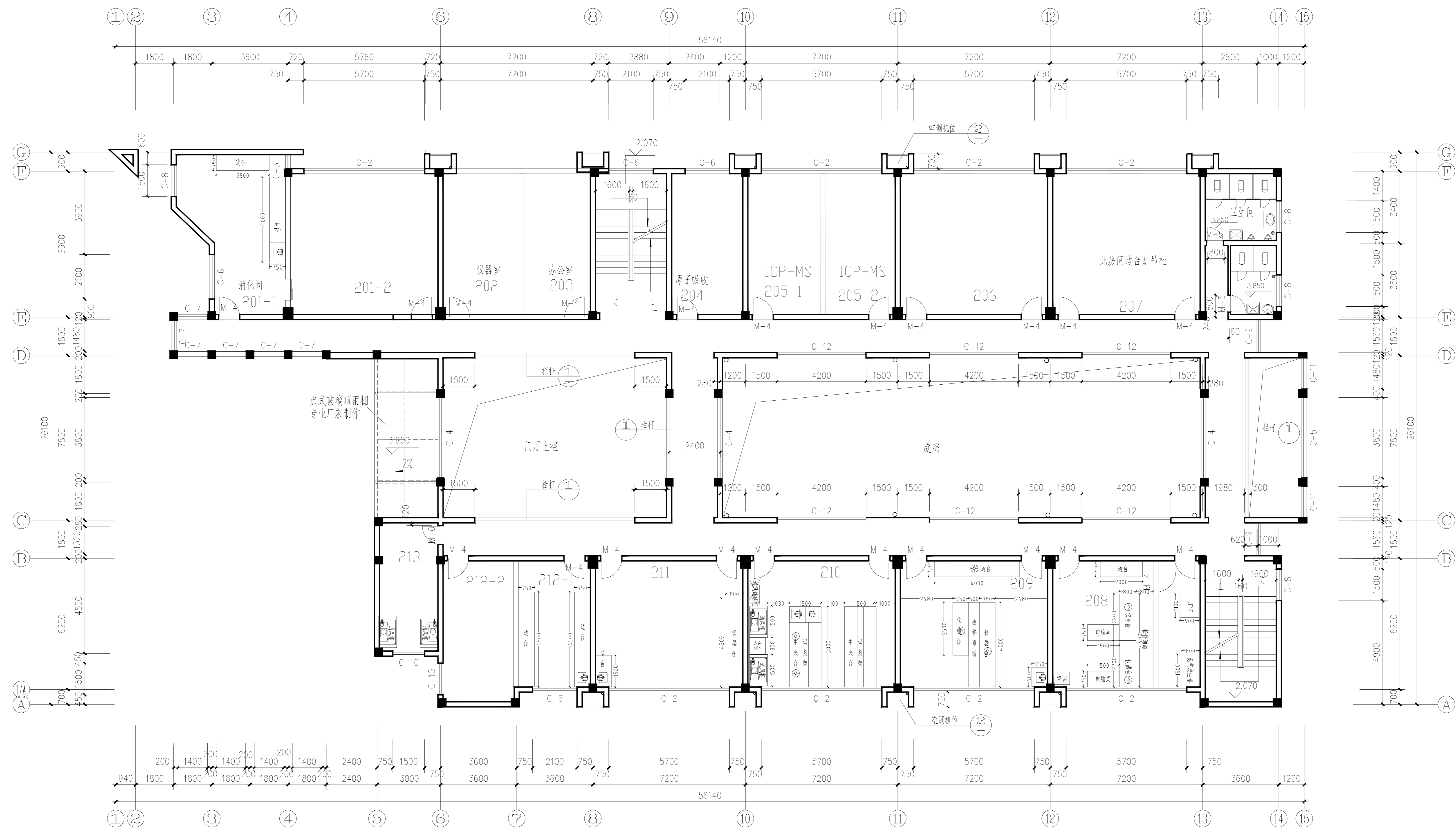
二层平面图1:100
